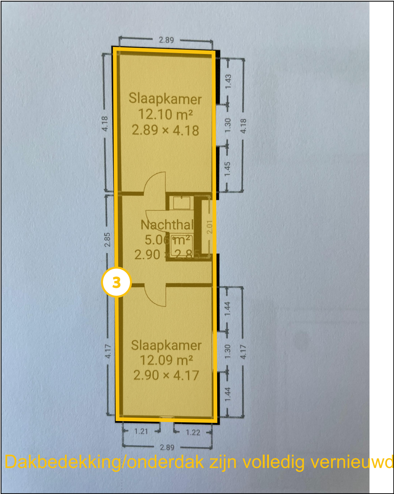
Legende van plan 1.3: Grondplan zolderverdiep
